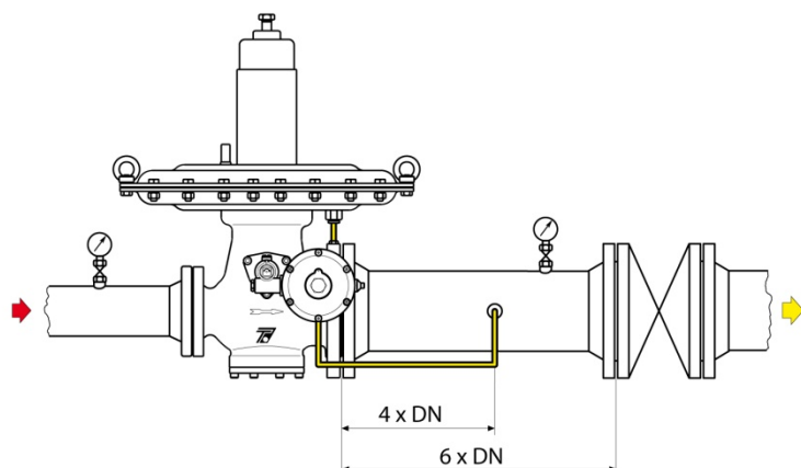
DN 25 - 65 С внутренним импульсным соединением
