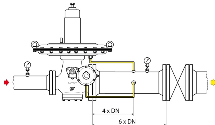
DN 80 - 100 Внешнее импульсное соединение
