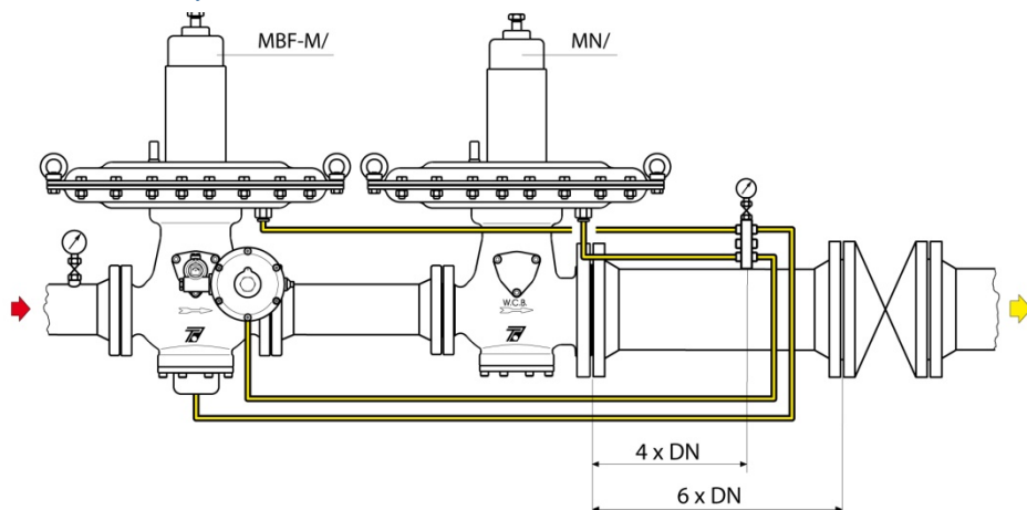
Внешнее импульсное соединение
