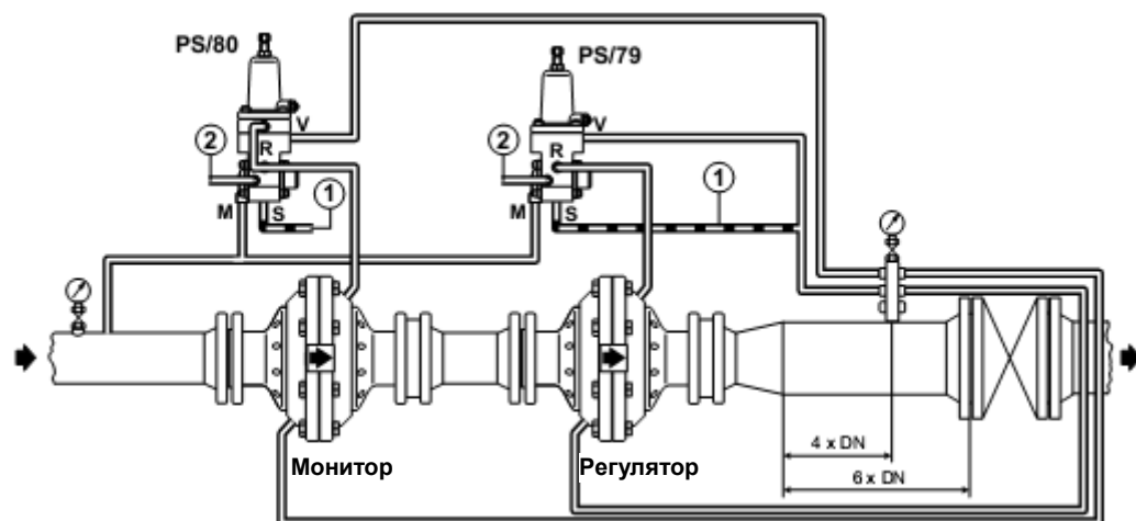
РЕГУЛЯТОР ТИПА FL И МОНИТОР С ПИЛОТОМАМИ PS/79 В PS/80
