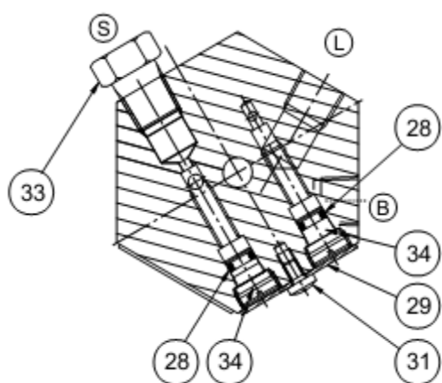
СЕЧЕНИЕ А-А
