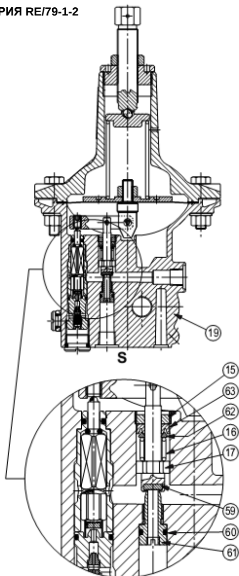
Рисунок 33. Пилоты серии PS/79-1, PS/79-2, RE/79-1 и RE/79-2 (продолжение)
