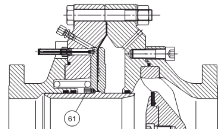
ДЕТАЛЬ FL-BP/150
