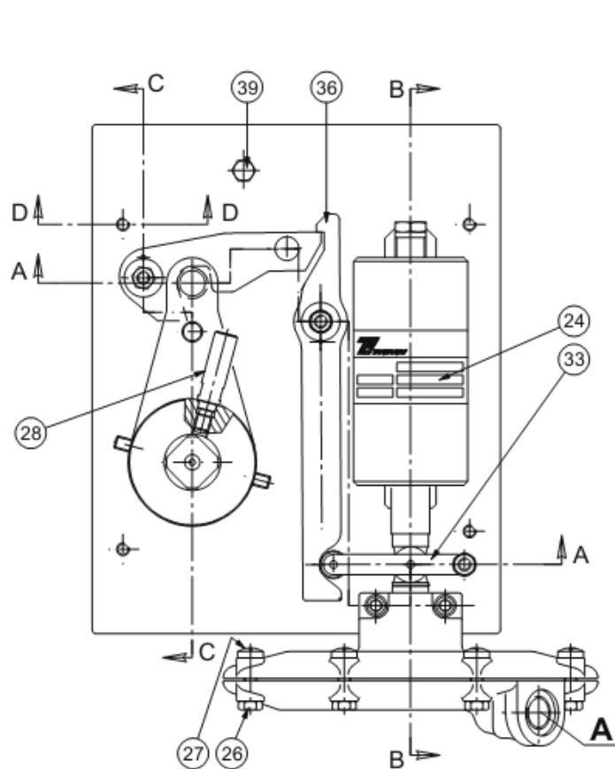
Рисунок 25. Пилот привода серии OS/80X (стандартная версия) (продолжение)
