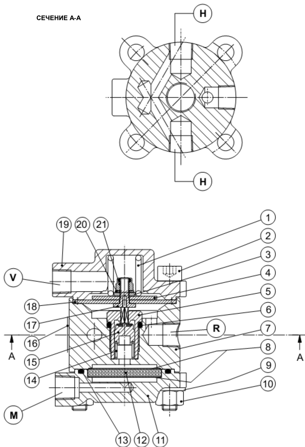
Соединения фильтра-стабилизатора SA/2
