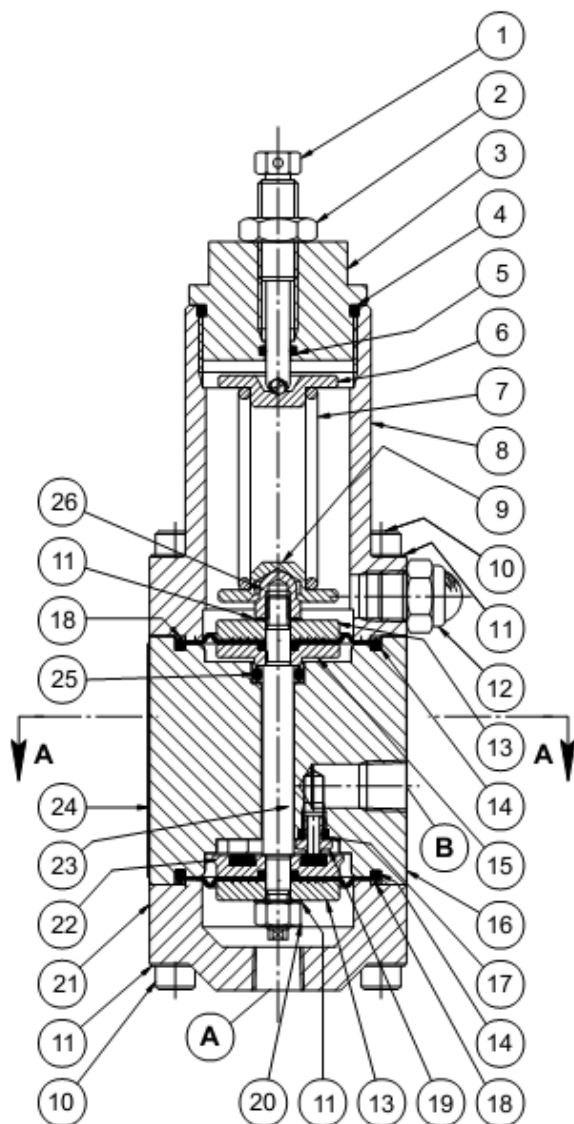
ПИЛОТ PRX/120 и PRX/125
