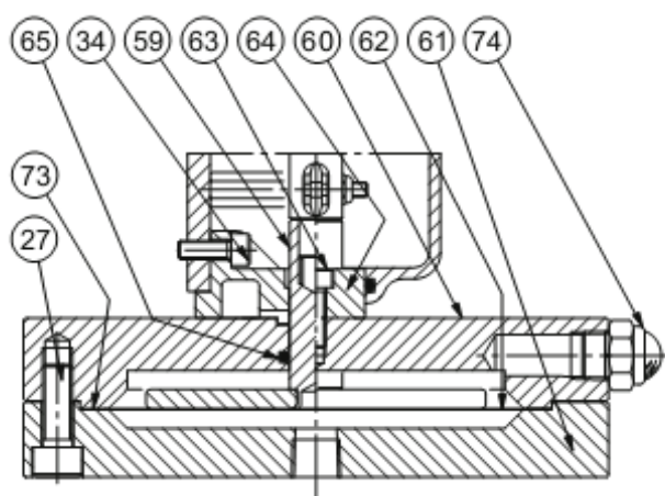
ДЕТАЛЬ OS/80X-BPA-D
