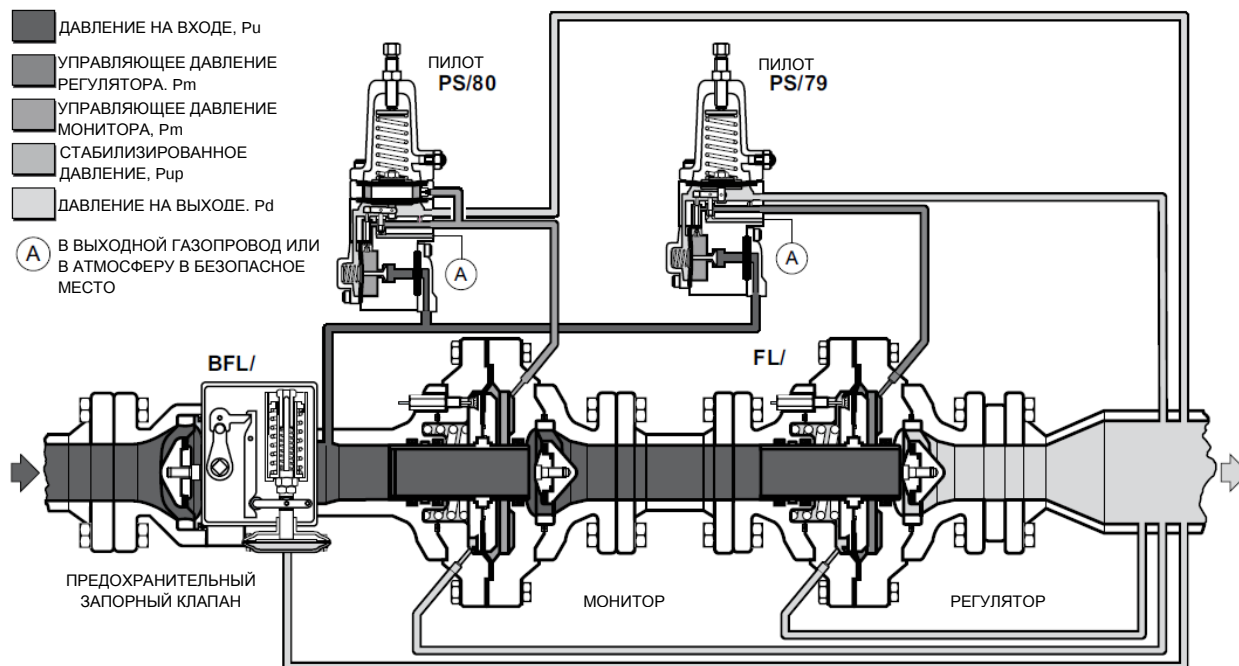
Рисунок 6 Схема работы типов BFL и FL
