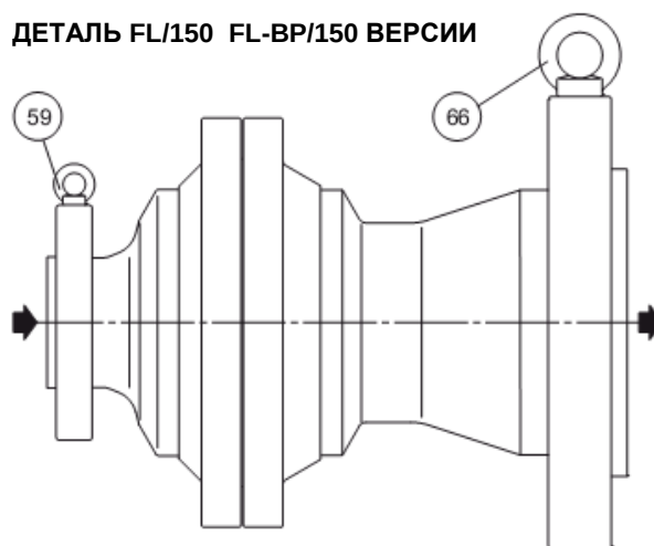
Рисунок 19. Различные версии регуляторов FL с DN 150
