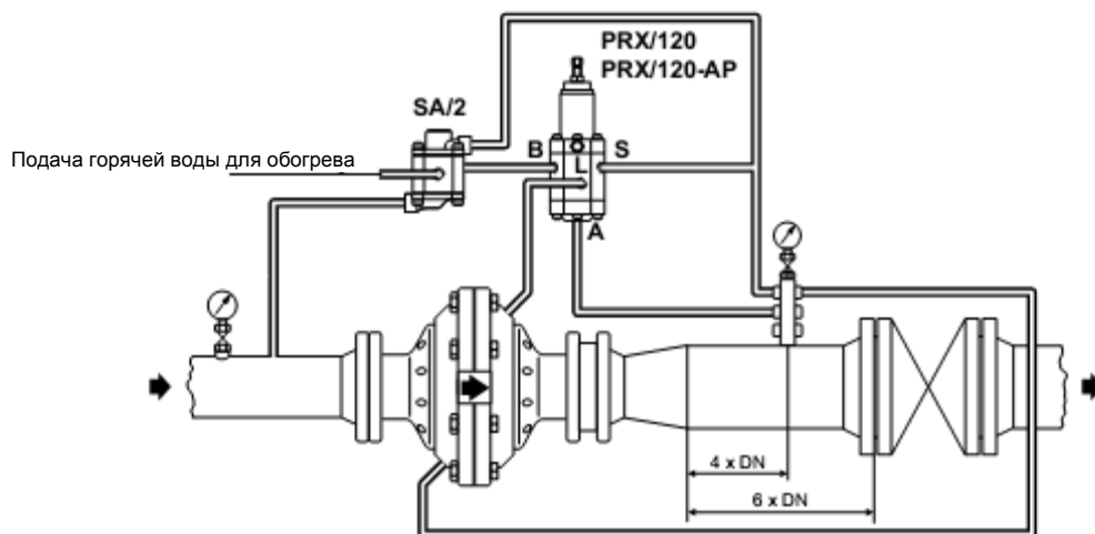
РЕГУЛЯТОР ТИПА FL С ПИЛОТОМ PRX/120 ИЛИ PRX/120-AP
