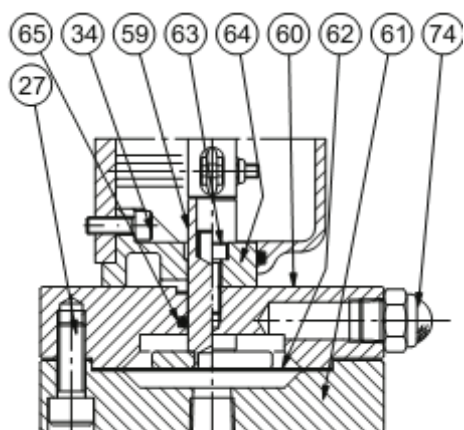
ДЕТАЛЬ OS/80X-APA-D
