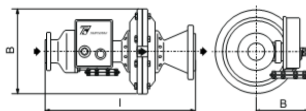
Рисунок 4. Размеры серии FL-BP
