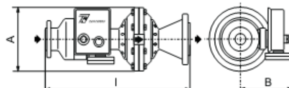
Рисунок 5. Размеры серии FL
