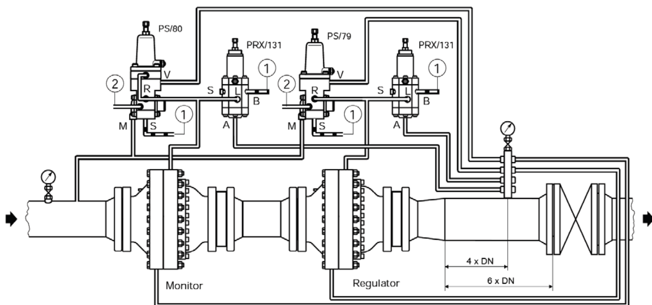
РЕГУЛЯТОР ТИПА FL/250 DN250 С ПИЛОТОМ PS/79, ПИЛОТОМ-УСКОРИТЕЛЕМ И МОНИТОР FL/250 DN250 С ПИЛОТОМ PS/80 И ПИЛОТОМ-УСКОРИТЕЛЕМ PRX/131
