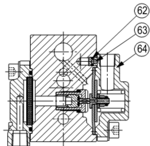
СЕРИЯ REO/79 И REO/80
