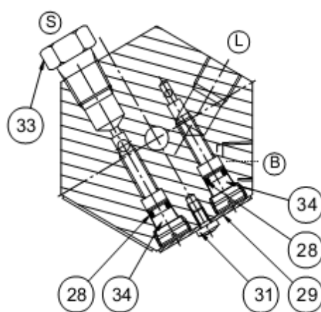
СЕЧЕНИЕ А-А
