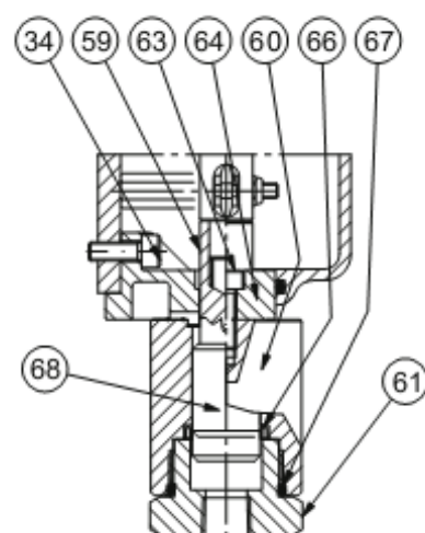
ДЕТАЛЬ OS/84X
