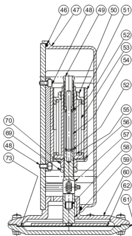
СЕЧЕНИЕ В-В 1-В
