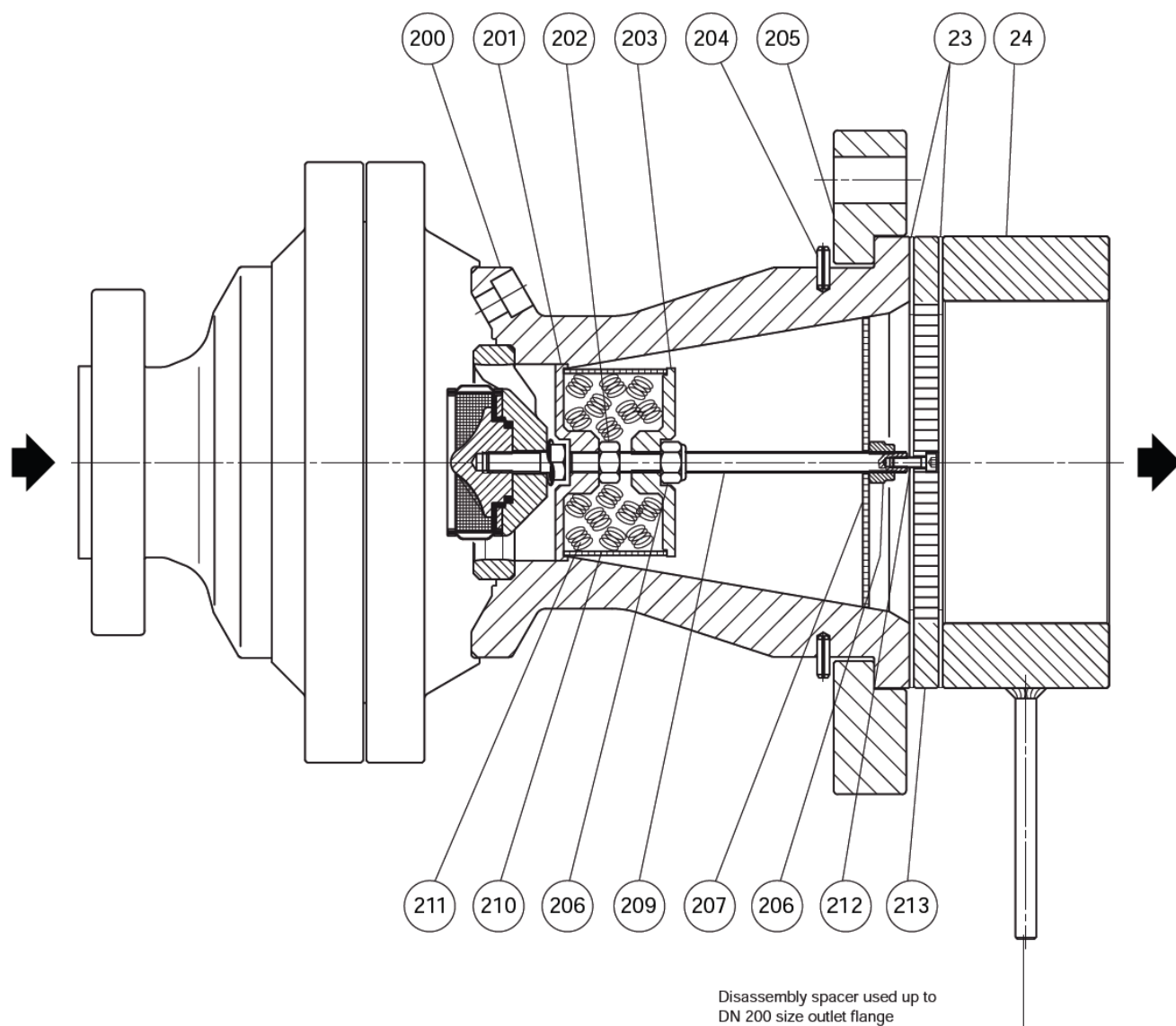
Рисунок 16. Регулятор FL с расширенным фланцем, версии SRS и SRS-R
