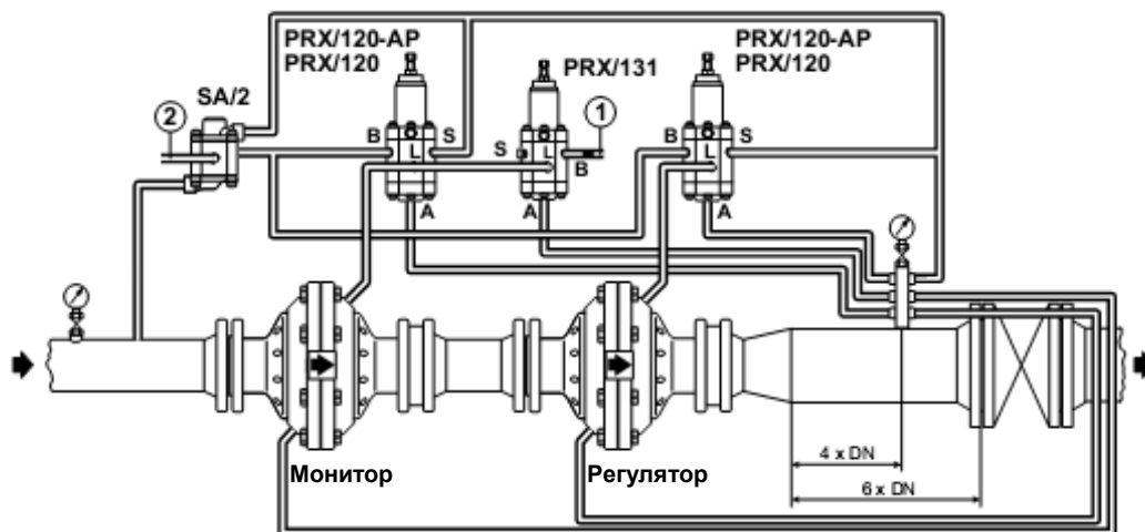
РЕГУЛЯТОР ТИПА FL И МОНИТОР С ПИЛОТОМАМИ PRX/120 И УСКОРИТЕЛЬНЫМ КЛАПАНОМ PRX/131
