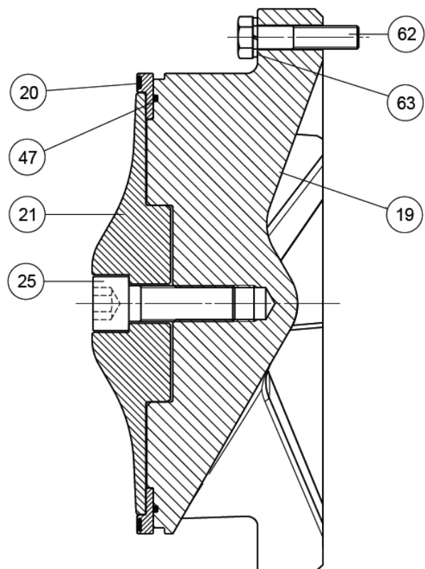
FL/250 DN250 БЕЗ ШУМОГЛУШИТЕЛЯ
