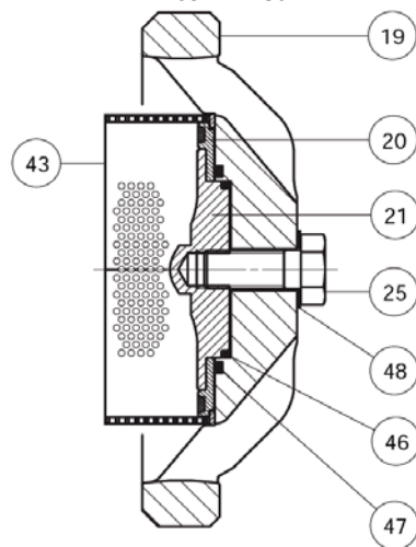
КРЕПЛЕНИЕ ПРОКЛАДКИ DN 65 - DN 80
