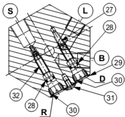
ПИЛОТ PRX/120 и PRX/125
