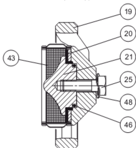
КРЕПЛЕНИЕ ПРОКЛАДКИ DN 25 - DN 50
