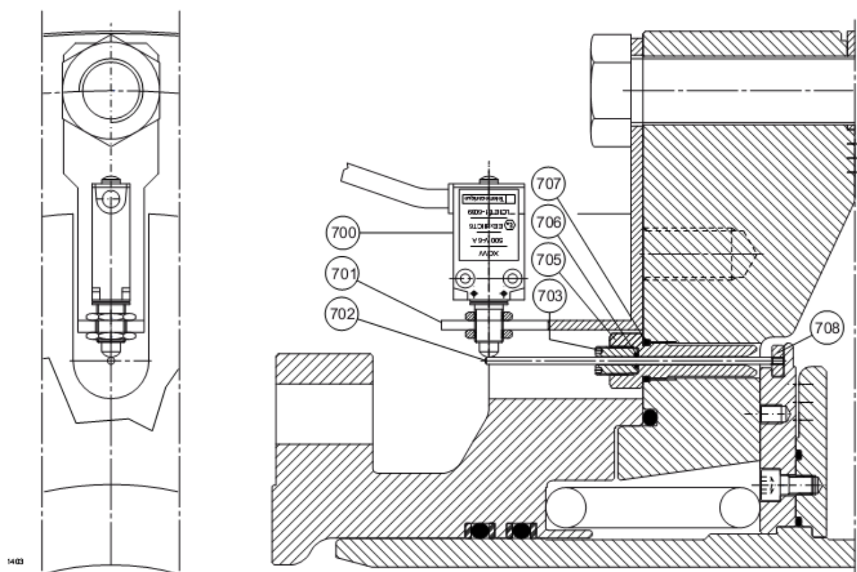
Рисунок 21. Регулятор FL с DN 200 с бесконтактным сигнализатором положения и микропереключателем
