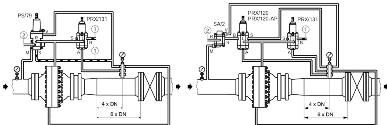
Регулятор давления FL/250 DN250 с пилотом PS/79 и пилотом-ускорителем PRX/131
