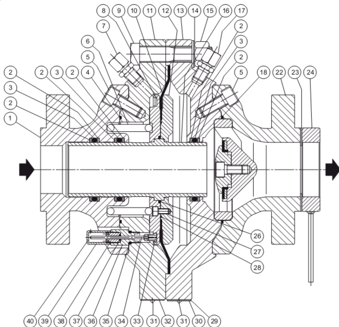
Рисунок 8. Регулятор FL DN 25-DN 150
