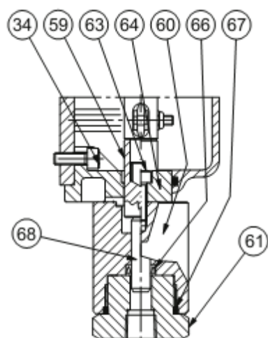
ДЕТАЛЬ OS/88X
