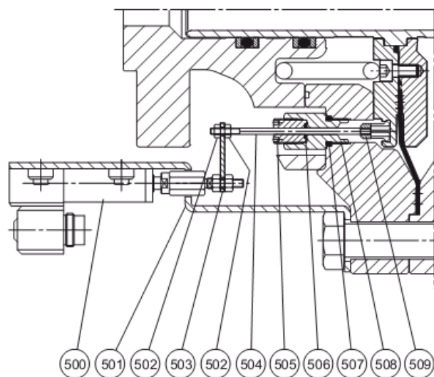
ВЕРСИЯ FL/ С ПРОПОРЦИОНАЛЬНЫМ ПЕРЕДАТЧИКОМ ХОДА
