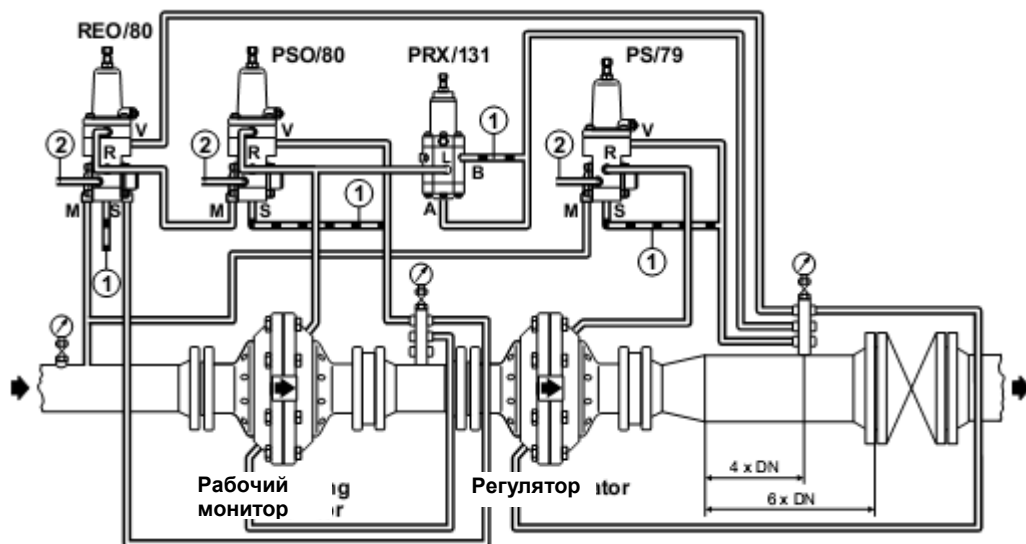
РЕГУЛЯТОР ТИПА FL И РАБОЧИЙ МОНИТОР С ПИЛОТОМ PS/79, PSO/80, REO/80 И УСКОРИТЕЛЬНЫМ КЛАПАНОМ PRX/131 ПОЯСНЕНИЕ:
