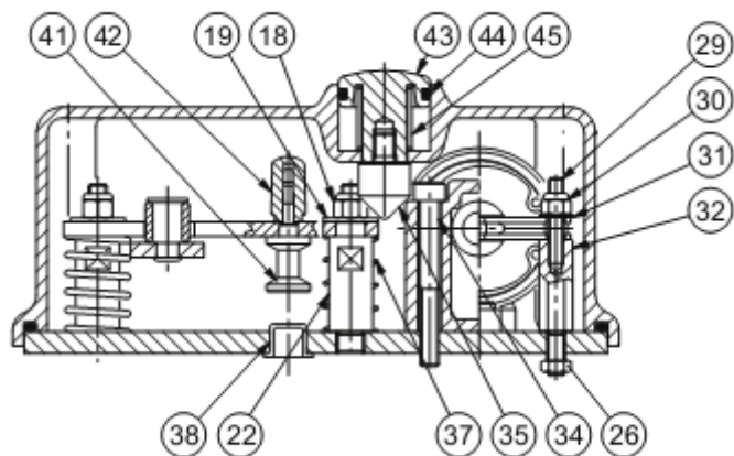
СЕЧЕНИЕ А-А
