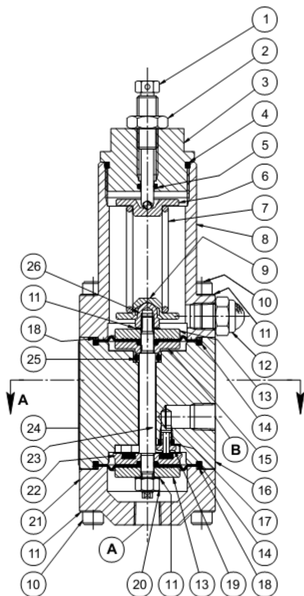
ПИЛОТ СЕРИИ PRX/181 В СБОРЕ
