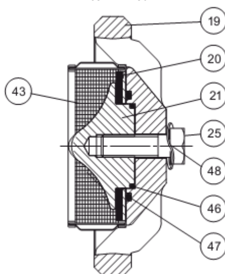
КРЕПЛЕНИЕ ПРОКЛАДКИ DN 65 - DN 150
