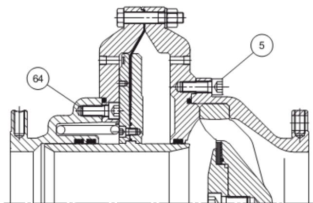
ДЕТАЛЬ FL/150 ANSI 300-600
