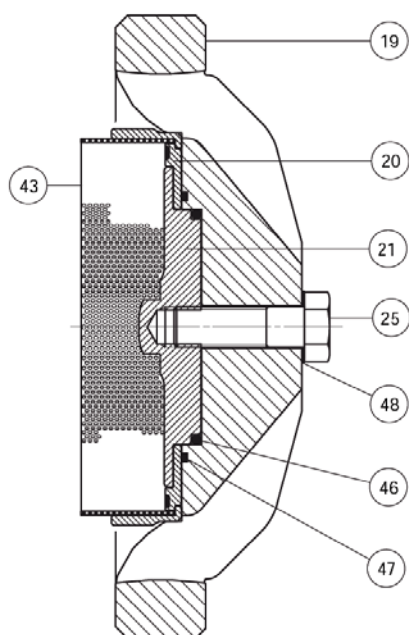
КРЕПЛЕНИЕ ПРОКЛАДКИ DN 100 - DN 150
