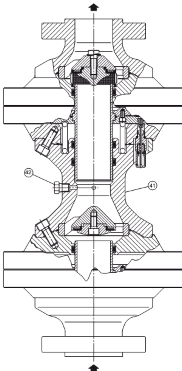
Рисунок 18. Регулятор MFL
