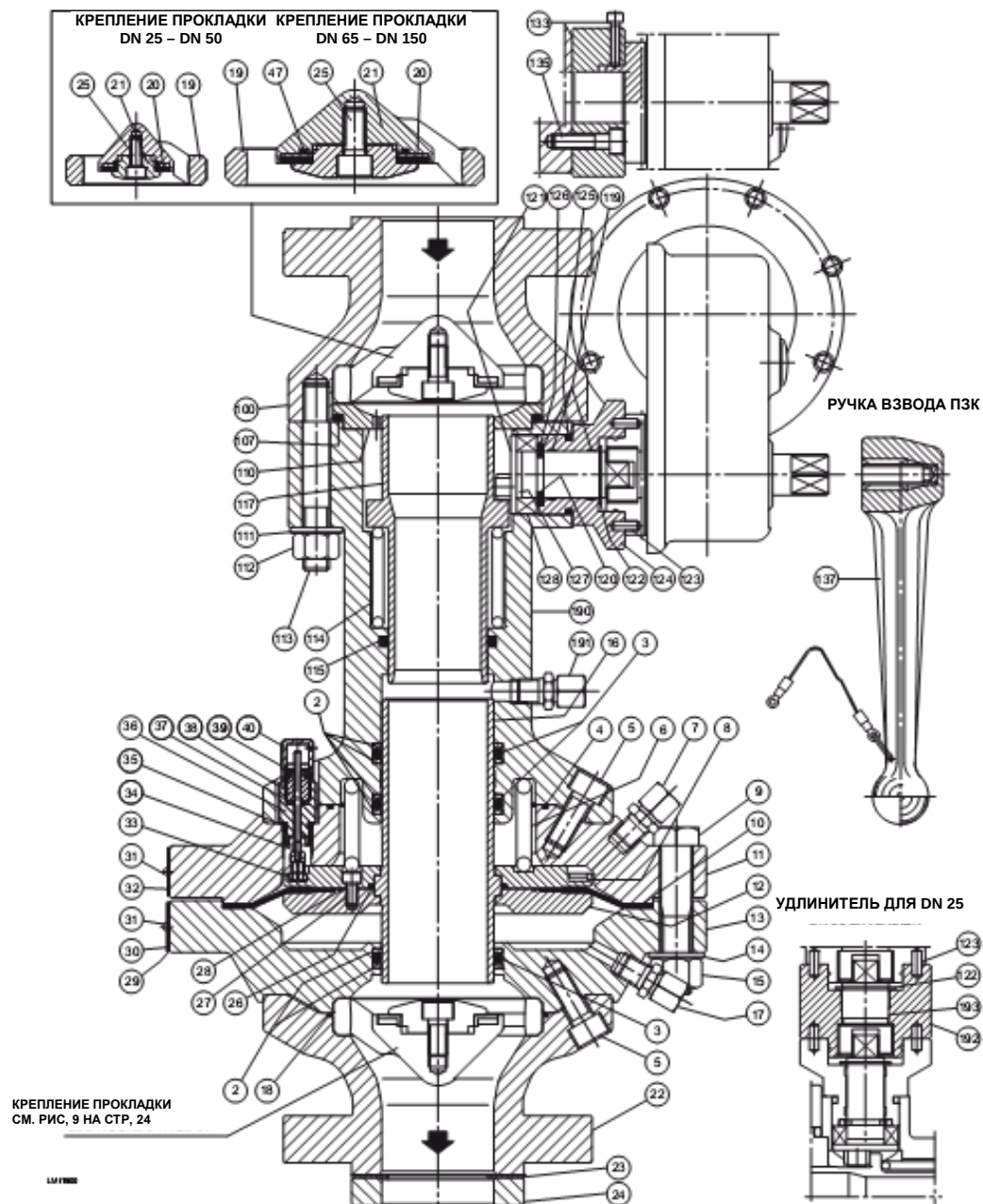
Рисунок 23. Регулятор BFL с предохранительным запорным клапаном
