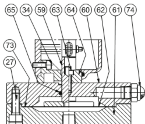
ДЕТАЛЬ OS/80X-MPA-D
