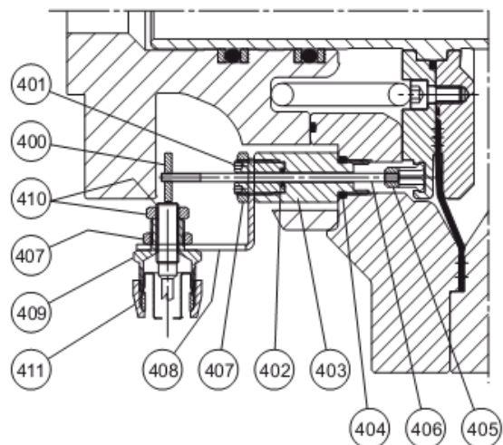
ВЕРСИЯ FL/ FL-BP/ С БЕСКОНТАКТНЫМ СИГНАЛИЗАТОРОМ ПОЛОЖЕНИЯ
