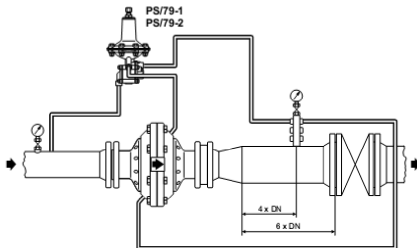
РЕГУЛЯТОР ТИПА FL-BP С ПИЛОТОМ PS/79-1-2
