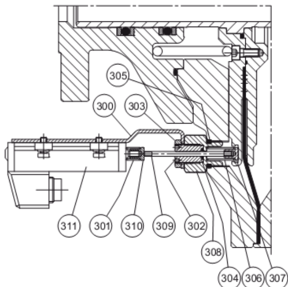
ВЕРСИЯ FL/ С ПРОПОРЦИОНАЛЬНЫМ ПЕРЕДАТЧИКОМ ХОДА
