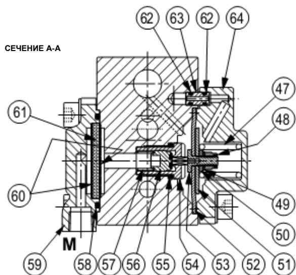
Рисунок 30. Пилоты серии PS/79, PS/80, RE/79 и RE/80
