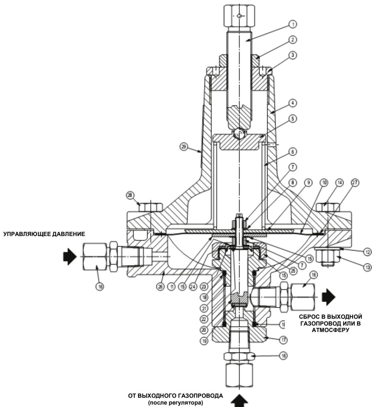
Рисунок 34. Ускорительный клапан типа V/31-1
