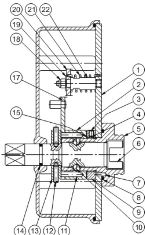
СЕЧЕНИЕ C-C
