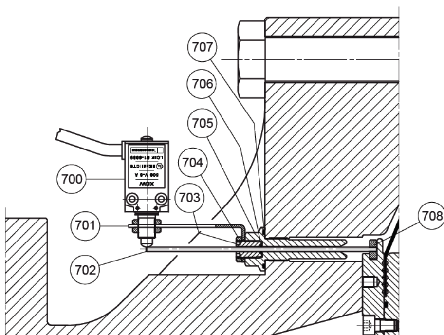
Рисунок 22. Регулятор FL с DN 250 с бесконтактным сигнализатором положения и микропереключателем
