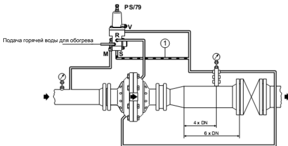
РЕГУЛЯТОР ТИПА FL С ПИЛОТОМ PS/79
