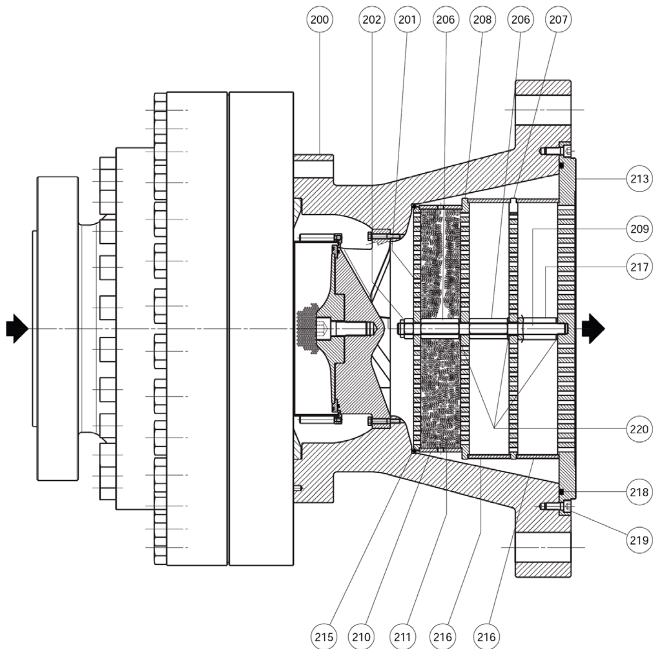
Рисунок 17. Регулятор FL с расширенным фланцем, версии SRSII
