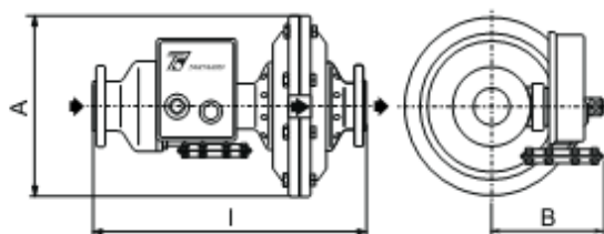
Рисунок 4. Размеры серии FL-BP
