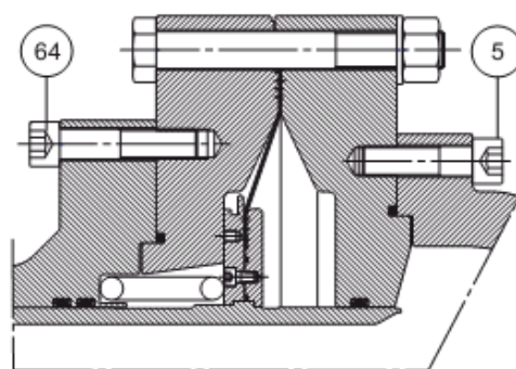
ДЕТАЛЬ FL/150 ANSI 300-600
