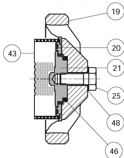
КРЕПЛЕНИЕ ПРОКЛАДКИ DN 25 - DN 50
