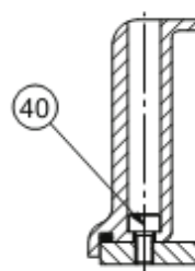
СЕЧЕНИЕ D-D
