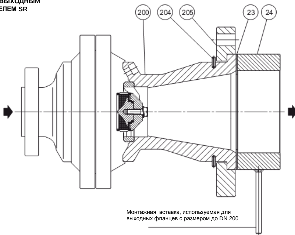
Рисунок 14. Версии регулятора FL с увеличенным выходным фланцем и увеличенным выходным фланцем с шумоглушителем SR
