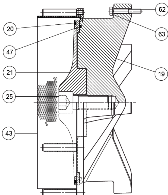
FL/200 DN200 И FL/250 DN250 С ШУМОГЛУШИТЕЛЕМ SRSII
