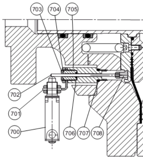
ВЕРСИЯ FL/ С МИКРОПЕРЕКЛЮЧАТЕЛЕМ
