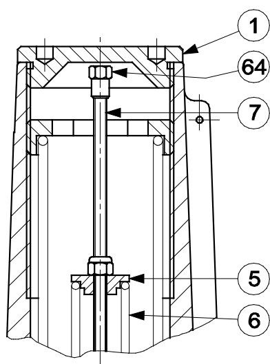
ДЕТАЛЬНЫЙ ЧЕРТЕЖ ВР (ВЕРСИЯ НА НИЗКОЕ ДАВЛЕНИЕ)
