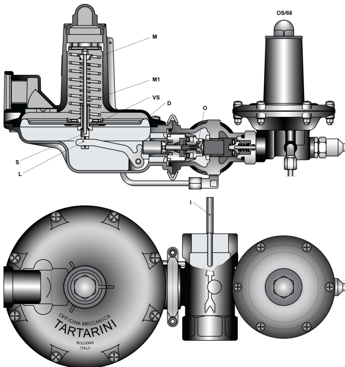
Рисунок 5. Схема работы регуляторов серии В/240
