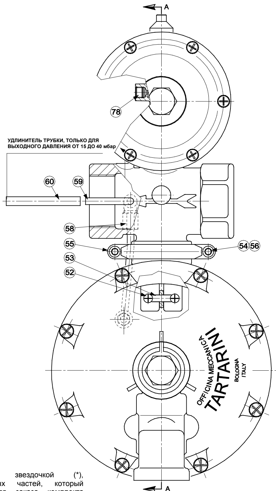
Рисунок 6. Регулятор серии В/240
