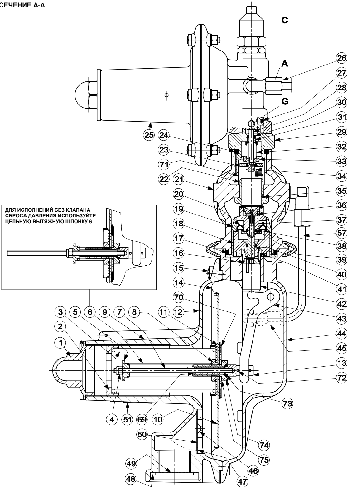
Рисунок 6. Регулятор серии В/240 (продолжение)
