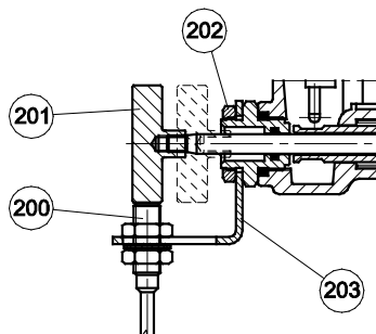
Рисунок 6. Регулятор серии А/140 (продолжение)
