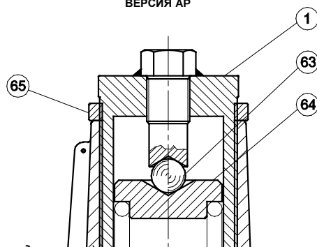
Рисунок 6. Регулятор серии А/140 (продолжение)
