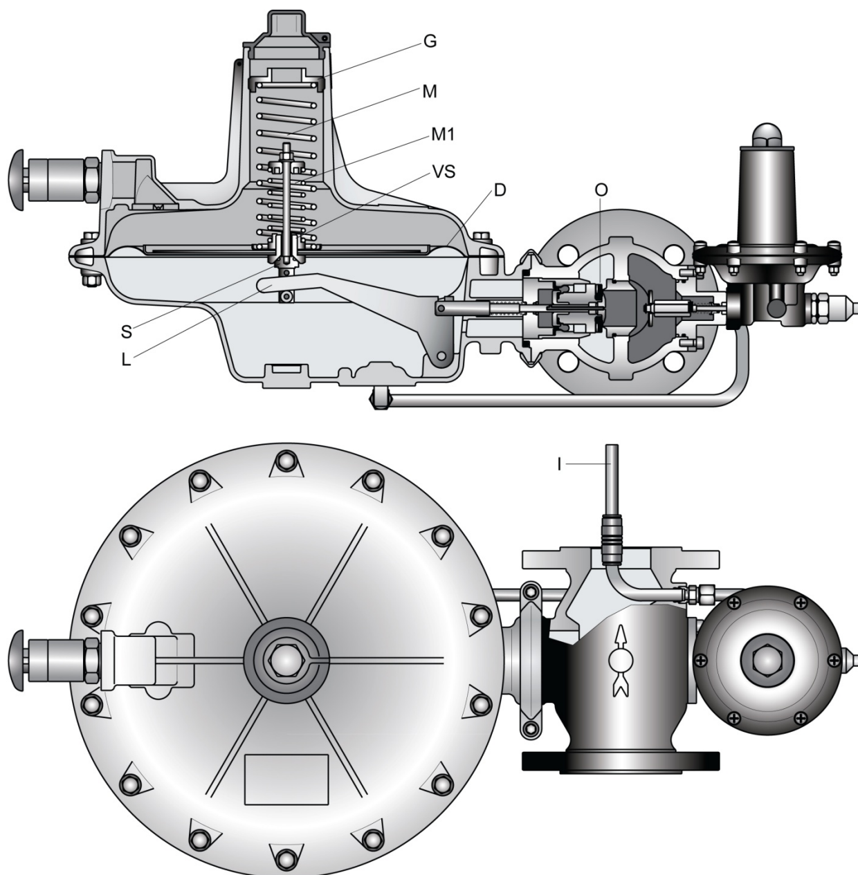
Рисунок 5. Схема работы регуляторов серии A/140
