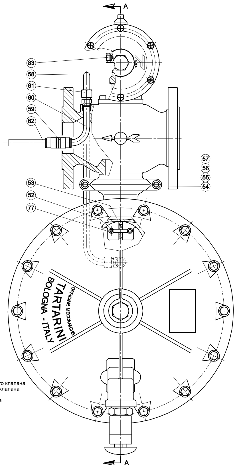
Рисунок 6. Регулятор серии A/140
